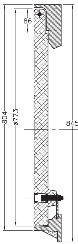
SECCION B-B
