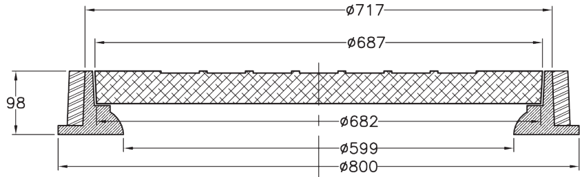
SECCION A-A
